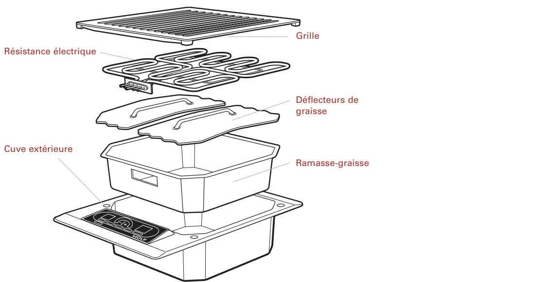
Assemblage du gril
